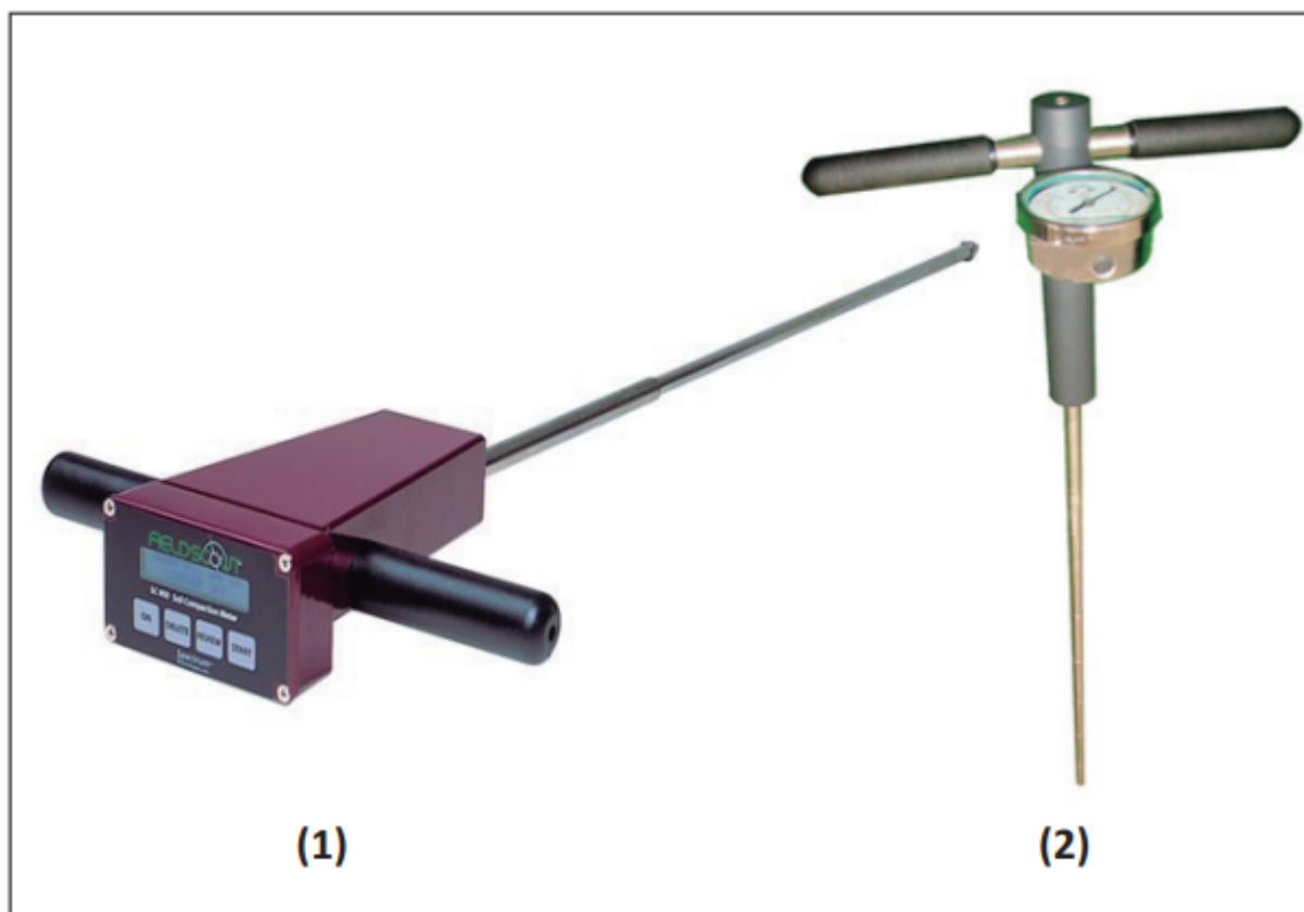
Foto 3. Penetrómetro de cono para el diagnóstico de capas compactadas del suelo (1) Penetrómetro digital, (2) penetrómetro analógico para medir la compactación.
